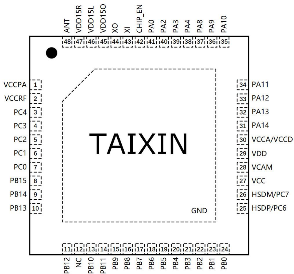
图1-4-2 TXW816-G0x QFN48封装脚位图
