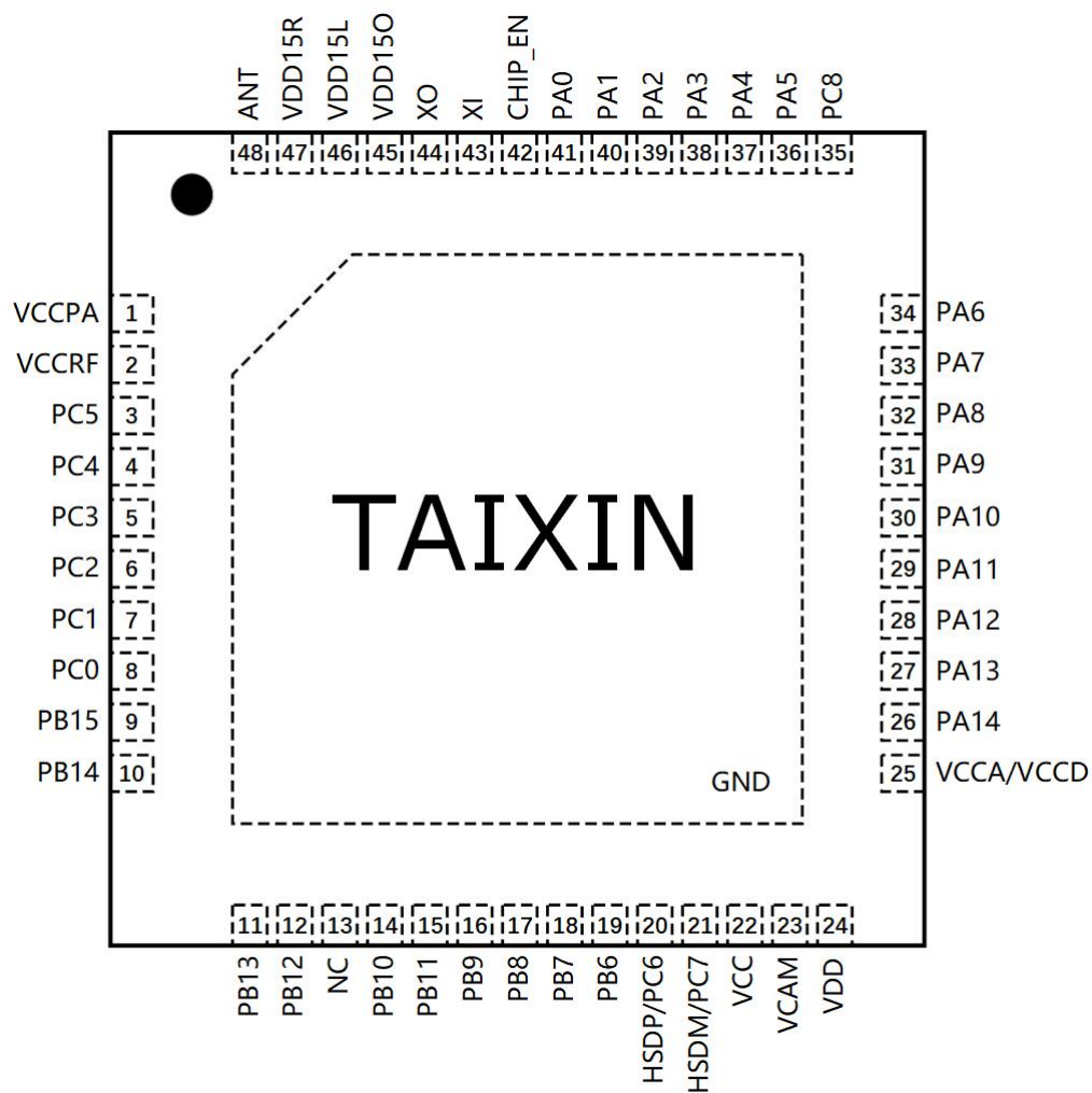
图1-4-1 TXW816-8xx QFN48封装脚位图
